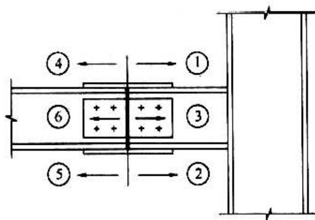
图3 工字梁节点施拧顺序
