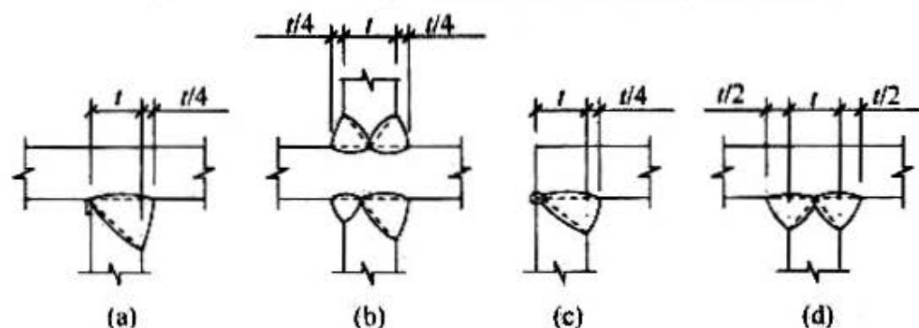
图 6.4.1 焊脚尺寸
