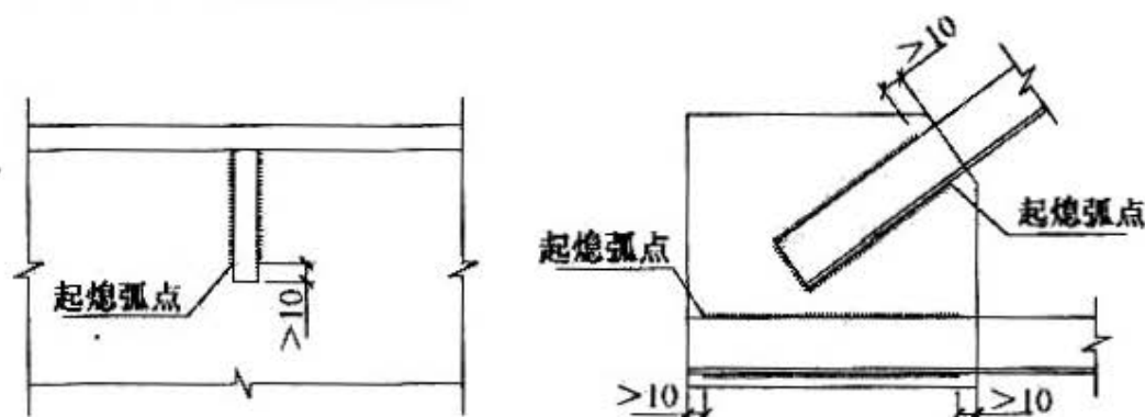
图 6.4.6 起熄弧点位置
