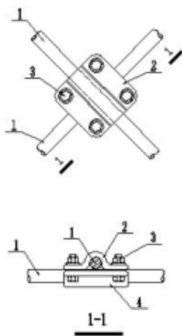
图 8.6.1-1 拉索的交叉连接（拉索连续）
