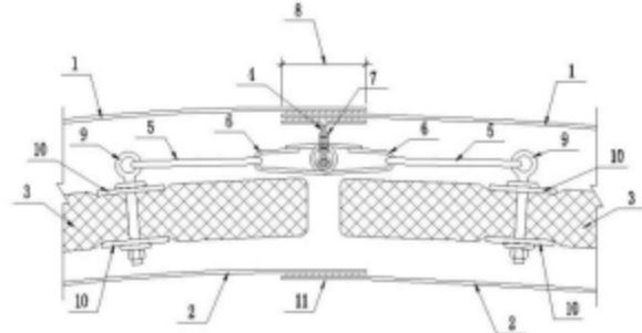
图 8.3.2-2 双层膜和保温材料在屋脊的连接
