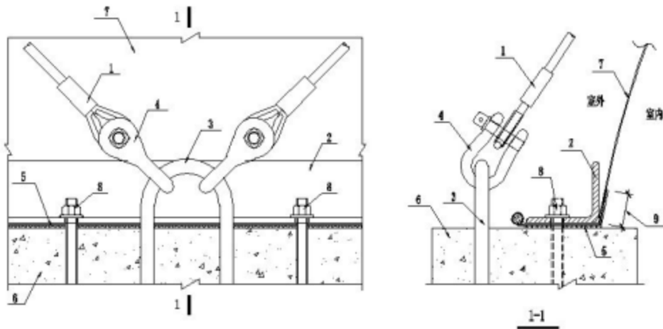
图 8.6.2-2 拉索与支承面的连接（拉索分股）
