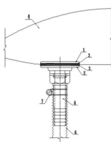
图 8.7.1 气枕单元与充气软管的连接 1—进气口上压盘；2—进气口下压盘；3—垫片；4—气枕； 5—进气口连接套；6—充气软管；7—膜盖
