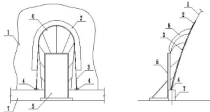
图 8.5.2-1 膜单元与气密门的连接（边索在软连接外）
