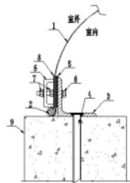
图 8.4.1-3 膜单元与支承面的连接（角钢）
