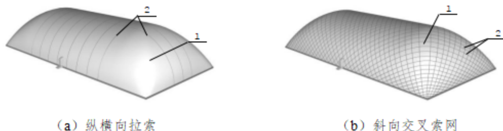
图 3.3.2 常用索网布置
