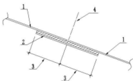
图 8.2.2-2 单层膜的对接连接
