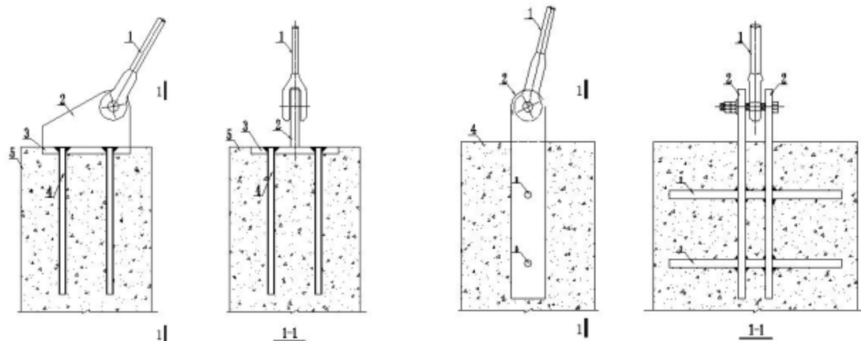
图 8.6.3-1 拉索与支承面连接（预埋钢加劲板） 1—拉索；2—耳板；3—钢板；4—锚筋；5—混凝土基础
