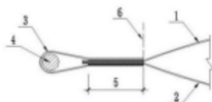
图 8.2.5 双层膜的收边连接
