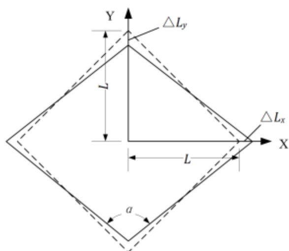
图 C.0.2-2 双轴剪切变形示意图
