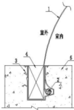
图 8.4.1-1 膜单元与支承面的连接（铝槽）
