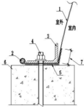
图 8.4.1-2 膜单元与支承面的连接（钢筋）
