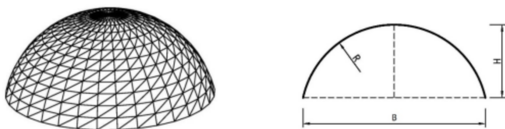
图 7.3.3-1 圆球形充气膜结构
